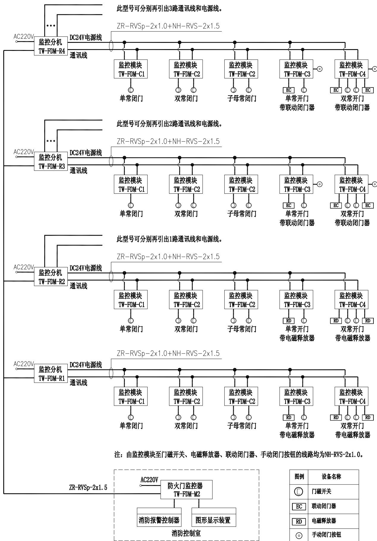
防火门监控系统示意图
